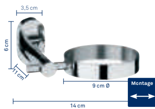
Föhnhalter Hair dryer holder Porte-sèche-cheveux
