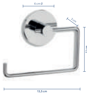
WC-Papierhalter Toilet paper holder Porte-rouleau papier toilette 1 4 24 ☒ 20153 4025457201530
